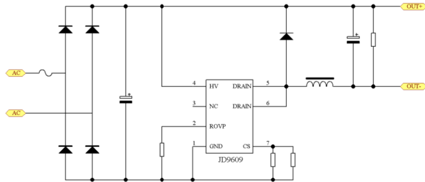
图 1 JD9609 典型应用图
