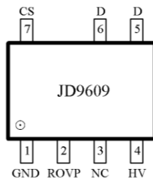
图 2 管脚封装图
