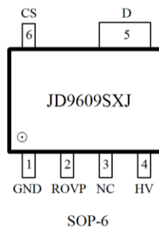
图 2 管脚封装图
