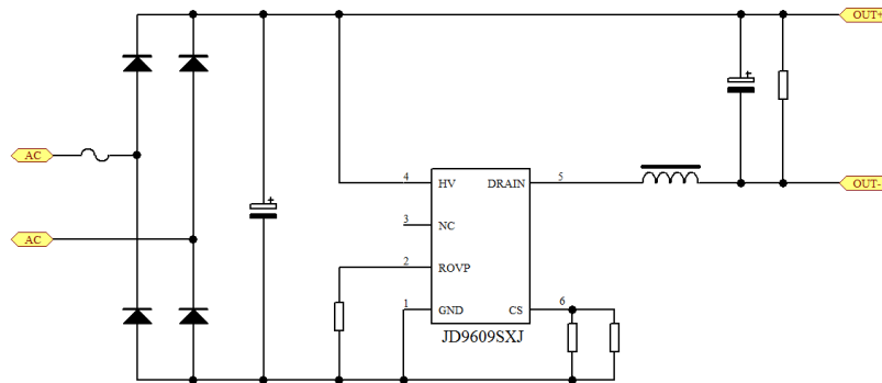
图 1 JD9609SXJ 典型应用图
