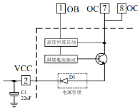
图 4 启动原理图
