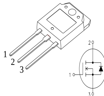
1 栅极(G) 2 漏极(D) 3 源极(S)
